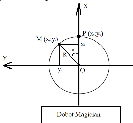
Рисунок 2. Окружность на координатной плоскости Dobot Magician
