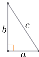
Рисунок 1. Прямоугольный треугольник: а и b – катеты, c – гипотенуза.
