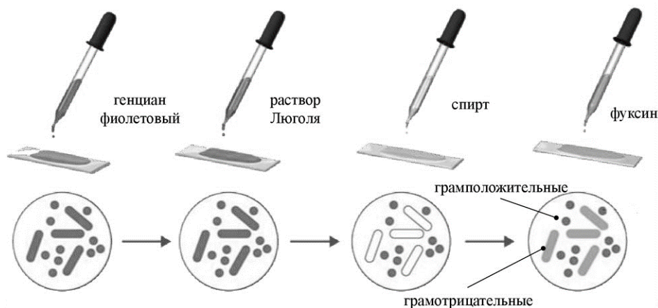
Рисунок 2. Схема окраски по Граму
