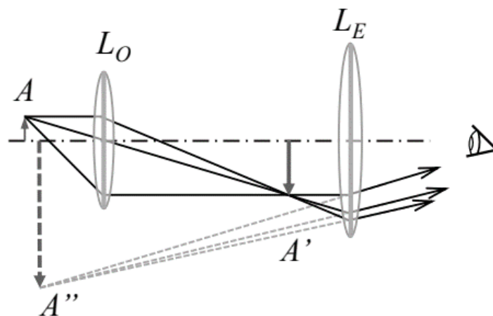
Рисунок 1. Ход лучей в двухлинзовом микроскопе. L_O – объектив, L_E – окуляр, A - предмет, A' – промежуточное действительное изображение, A'' – мнимое изображение, наблюдаемое через окуляр
